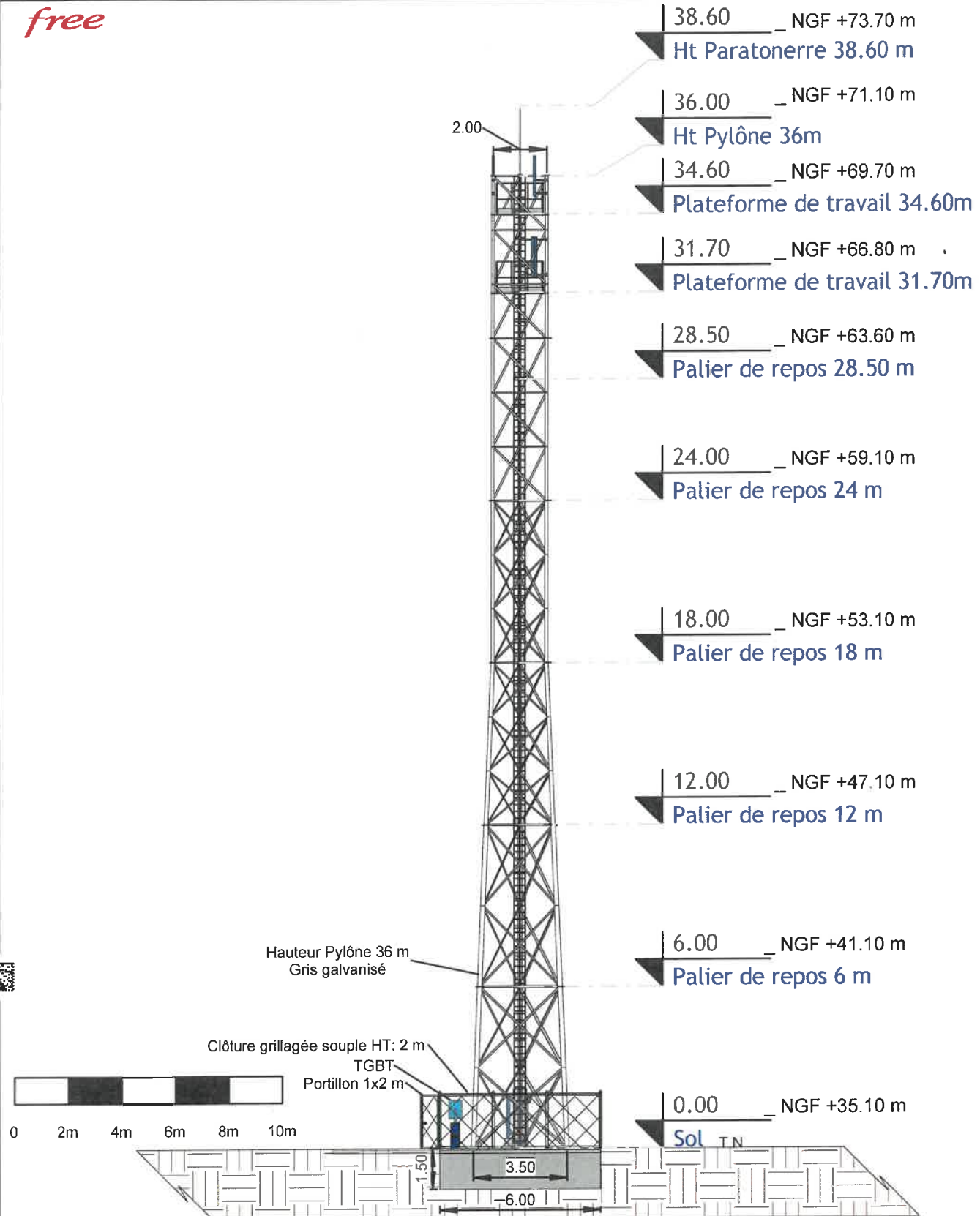
FREE-Elévation Sud-Pylône
